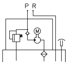
Diagram 油路圖
