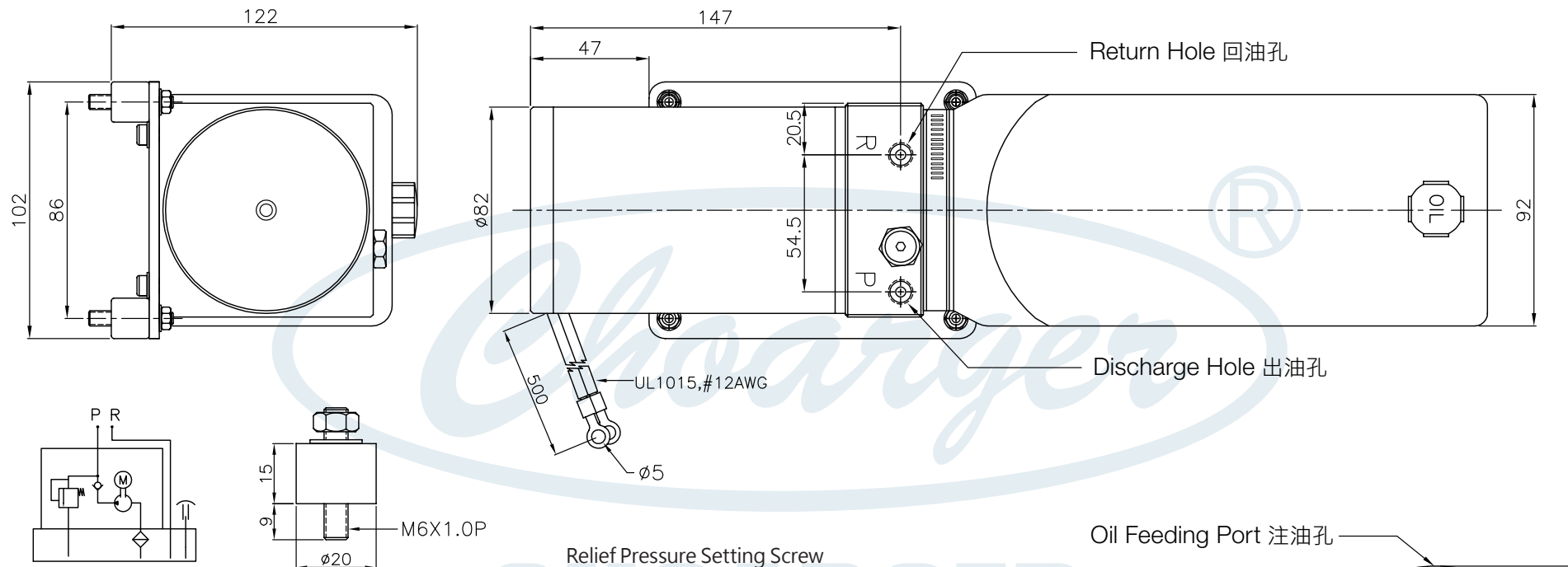
Diagram 油路圖
