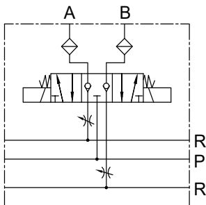
液壓迴路 Hydraulic Circuit
