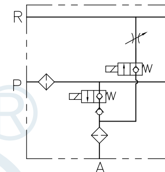
Diagram 油路圖
