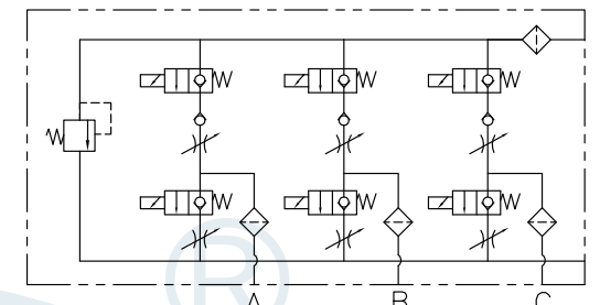
Diagram 油路圖
