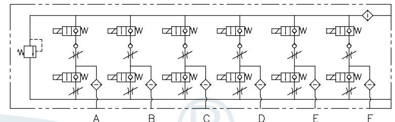
Diagram 油路圖
